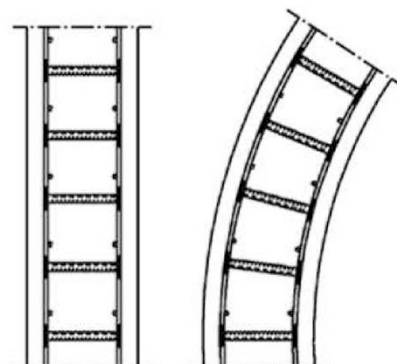
Beispiel 8: vertikale Plattenbauteile, Wand gerade, Wand gekrümmt
