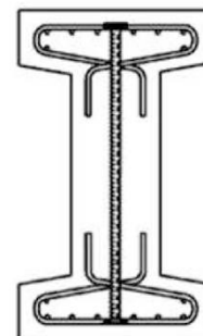
Beispiel 5: I - Träger
