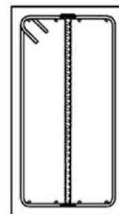
Beispiel 6: Kompaktquer- schnitt ( Balken bzw. Plattenbalken )
