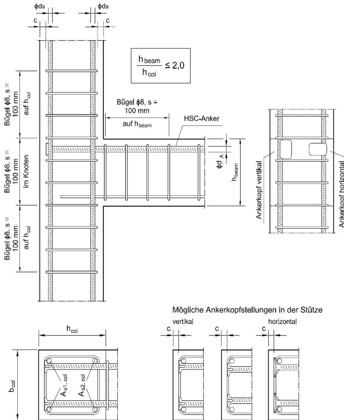
Abbildung 1: Bewehrungsführung, Beispiel
