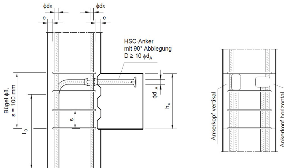
Abbildung 9: Bewehrungsführung von um 90^\circ nach unten abgebogenen HSC-Ankern in der Stütze, Beispiel
