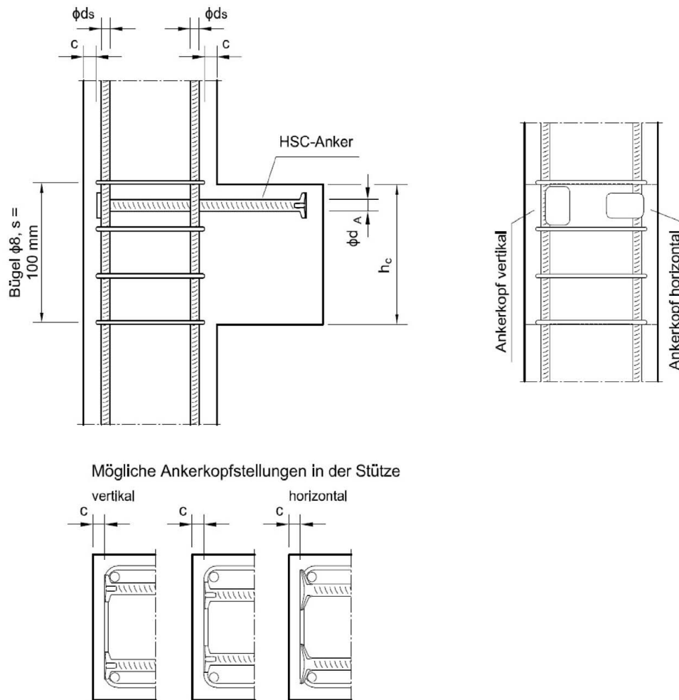
Abbildung 8: Bewehrungsführung in der Stütze, Beispiel
