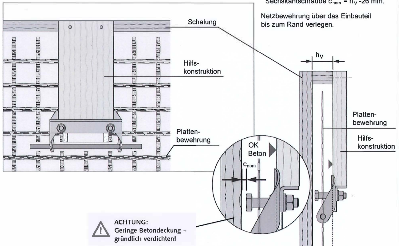
A2 Hilfskonstruktion an Schalung befestigen. Planmäßige Betondeckung unter Sechskantschraube c_{nom} = h_v - 26 mm.
