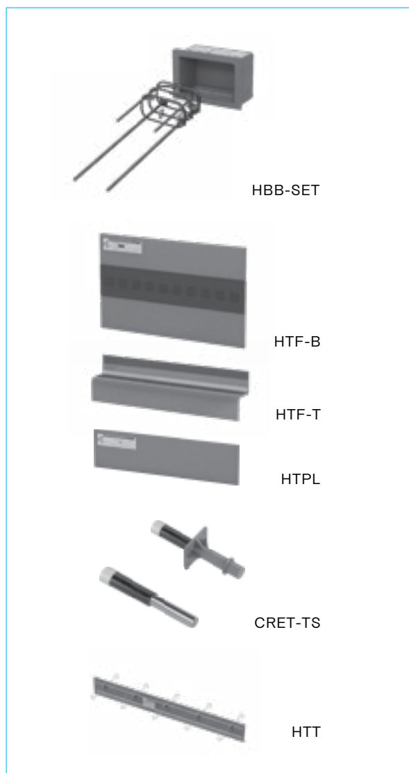
Prvky tlumení kročejového hluku
