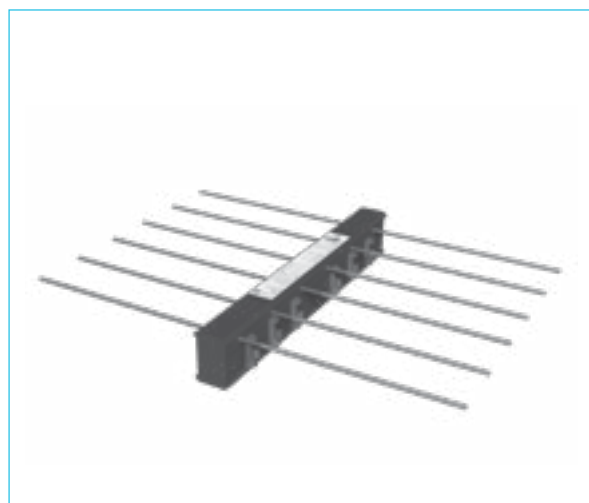
Balkónové izolační nosníky
