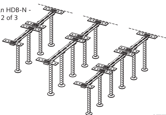
Figuur 2: De ponswapeningselementen worden van boven door de reeds aanwezige bovenwapening gestoken
